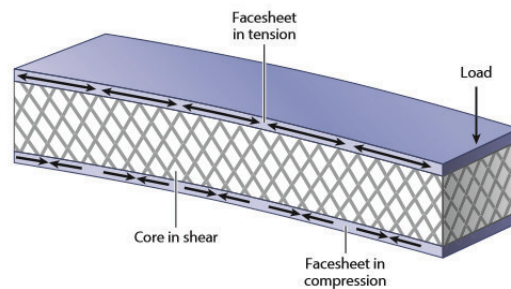
Figura 1. Viga tipo sándwich (Schaedler &amp; Carter, 2016)
